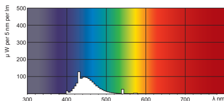
Lichtfarbe TL-D /180
