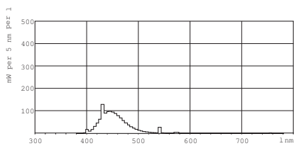
Lightcolor TL-D /180
