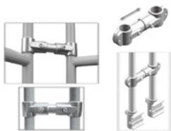
Best.-Nr. 8070287T GUIL TMU-06 Verbinder für Geländer
