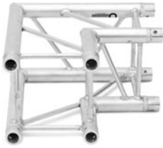
ALUTRUSS QUADLOCK QL-ET34 C-21 2-Wege-Ecke 90° Best.-Nr. 60306780.....5,8 kg
