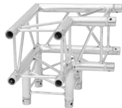
ALUTRUSS QUADLOCK 6082L-30 3-Wege-Ecke 90° Best.-Nr. 60306565.....8 kg
