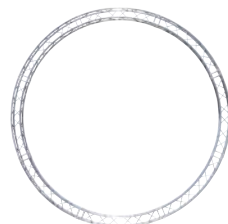
ALUTRUSS QUADLOCK 6082 Vollkreis (innen) Best.-Nr. 60306700..... 2 m Best.-Nr. 60306702..... 3 m Best.-Nr. 60306704..... 4 m Best.-Nr. 60306706..... 5 m Best.-Nr. 60306708..... 6 m
