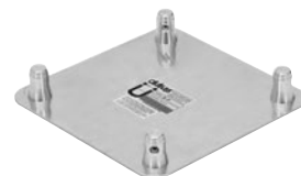
ALUTRUSS QUADLOCK Endplatte QQG-Konus Male Best.-Nr. 6030299A Best.-Nr. 6030299B..... mit Verbinderset
