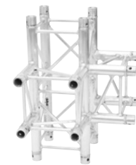
Best.-Nr. 60306580 ALUTRUSS QUADLOCK 6082T-42 4-Wege-T-Stück
