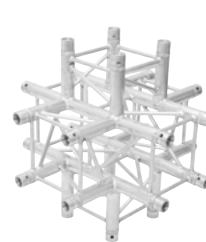
Best.-Nr. 60306590 ALUTRUSS QUADLOCK 6082C-61 6-Wege-Kreuzstück
