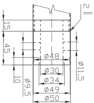
DETAIL A: SCALE 1:2
