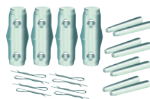
Best.-Nr. 60302895 ALUTRUSS QUADLOCK Satz Verb.konus/Zapfen/Splint QUADLOCK Satz
