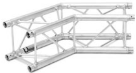
ALUTRUSS DECOLOCK DQ4-PAC23 2-Weg Ecke 135° Best.-Nr. 60301738.....2,4 kg
