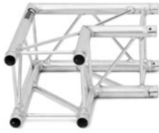
ALUTRUSS DECOLOCK DQ4-PAC21 2-Weg Ecke 90° Best.-Nr. 60301734.....4,6 kg
