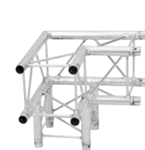
Best.-Nr. 60301744 ALUTRUSS DECOLOCK DQ4-PAL30 3-Weg Ecke 90°
