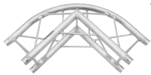
ALUTRUSS DECOLOCK DQ3-PAC24R 2-Weg Ecke 90° Best.-Nr. 60301675.....3,4 kg
