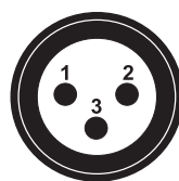
DMX-Eingang XLR-Einbaustecker:
