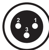
DMX-Ausgang XLR-Einbaubuchse:
