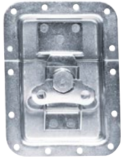
Best.-Nr. 30000400..... groß in Schale Best.-Nr. 30000600..... klein in Schale ROADINGER Butterfly-Schloss groß in Schale • Material: Stahl, verzinkt • Gewicht: ca. 460 g • Befestigungslöcher: D=5,1 mm
