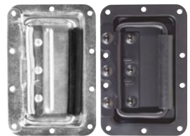
Best.-Nr. 30000900..... zink Best.-Nr. 30000920..... schwarz ROADINGER Case-Klappgriff • Klappgriff • Gewicht ca. 350 g • Ausschnitt 130 x 73 mm • Befestigungslöcher: D=5,0 mm
