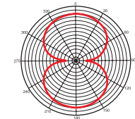
Richtcharakteristik (Acht) bei 1 kHz
