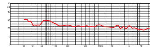
Frequenzgang (Acht)
