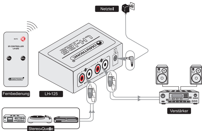
Abb. 4-1 Anschlussbeispiel
