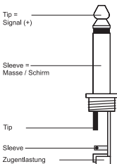
Unsymmetrische Betriebsart mit 6,35-mm-Mono-Klinkestecker
