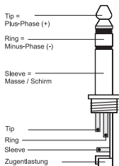
Symmetrische Betriebsart mit 6,35-mm-Stereo-Klinkestecker
